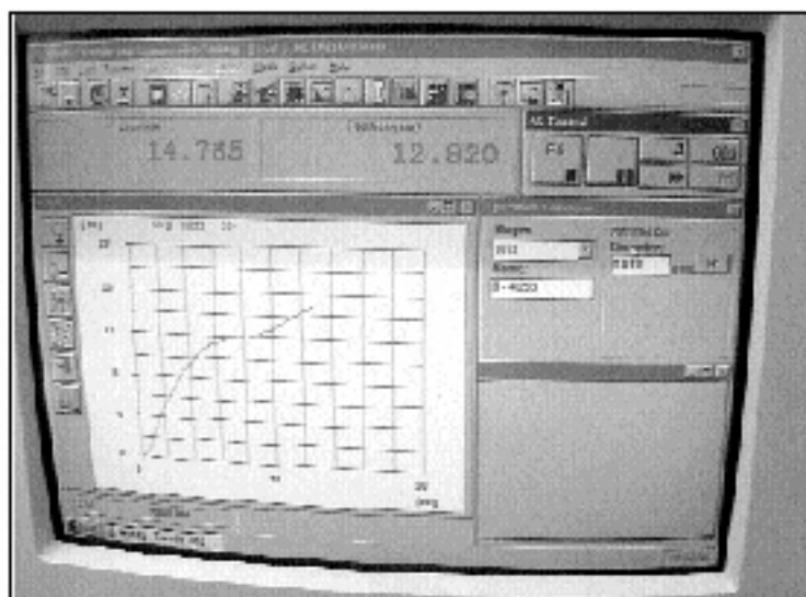
Vista en representación gráfica de aumento de aplicación de carga hasta alcanzar punto de inflexión de dicha carga (Zaké). "Carga aplicada supera resistencia a momento torsor del acople" Referencia Gráfico 3 = 3522 Nm. Resistencia Mt real obtenido Referencia Gráfico 4 = 3966 Nm. Resistencia Mt real obtenido
