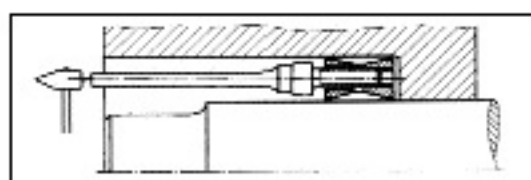
Figura 18: Aflojamiento del cono posterior Si el cono posterior se afloja, pulse ligeramente las cabezas de los tornillos hacia que está saliendo.
