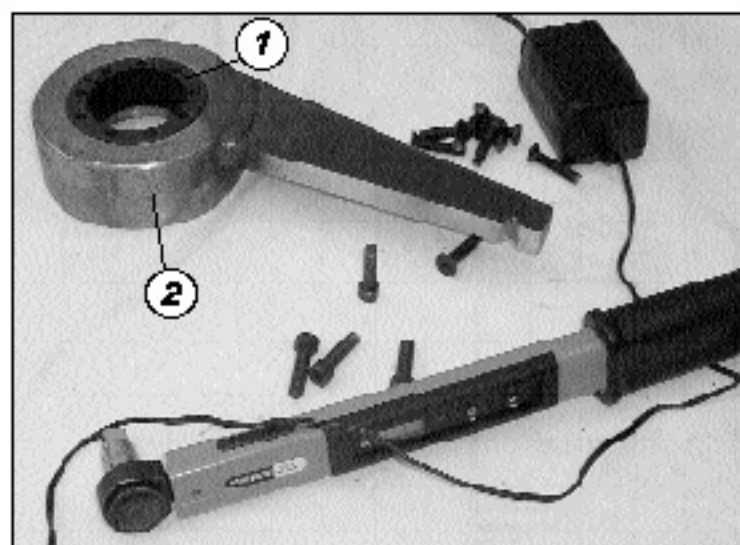
Ensamble de acople Blokear en alojamiento de maza del dispositivo de ensayo. Torquímetro digital utilizado para calibrar cupla de ajuste (Mb) indicada en tabla.
