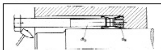
Figura 19: Aflojamiento del cono frontal Si el cono frontal se afloja, extraiga los 3 tornillos cromados en zinc para liberar las roscas ( d_1 ) del cono frontal. Inserte los tornillos o varis las roscadas correspondientes (ver herramientas de extracción) y pulse ligeramente hacia afuera para liberar el cono frontal. Las roscas extraíbles solo tienen de 3 a 5 filetes efectivos; no son adecuadas para realizar fuerza de extracción potente y solo deberán utilizarse para extraer el acople BLOKEAR BLK 200 EN CASO DE ENGRANE.
