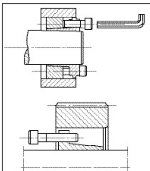
Figura 2: Procedimiento de desmontaje
